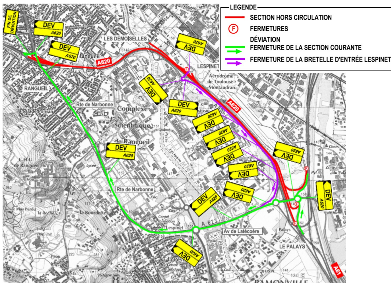
Figure 7 : Plan de déviation lors d'une fermeture du périphérique intérieur Palays - Rangueil
